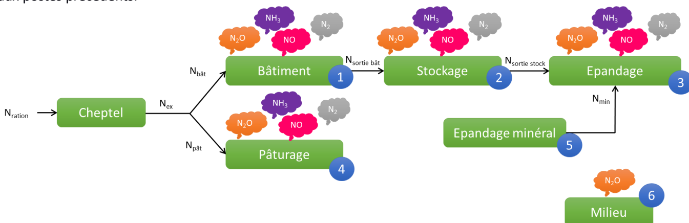
Figure 9 : Principe du calcul des émissions de gaz azotés sur les différents postes, à partir de l'azote ingéré via la ration alimentaire des animaux
